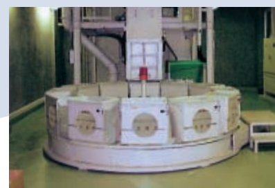
ロータリーバケット 圧縮・成形品の専用バケットは自動的に交換されるため連続処理が可能です。
