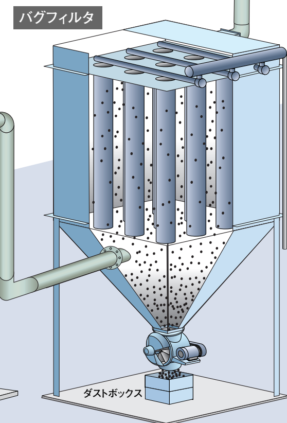
バグフィルタ へパフィルタ等の組合せで室内循環が可能となり空調エネルギーが効率的に活用出来ます。
