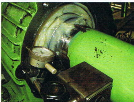
ベアリング交換後、軸受け芯だし調整
