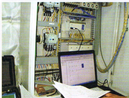
制御盤ソフト点検例
